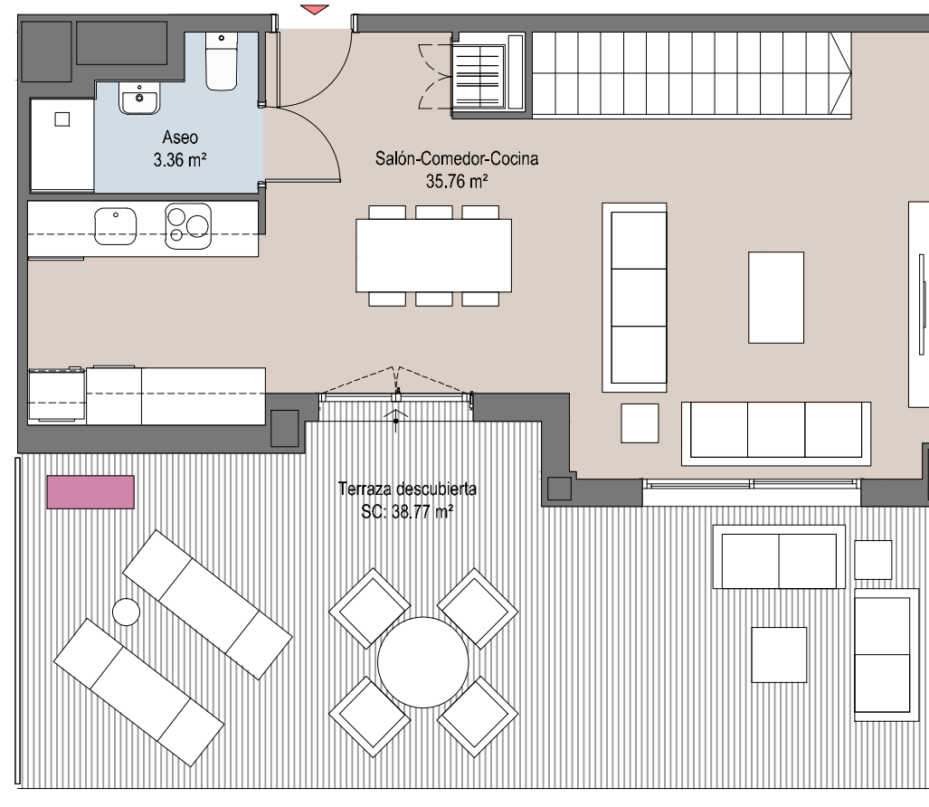
Planta 5 a
